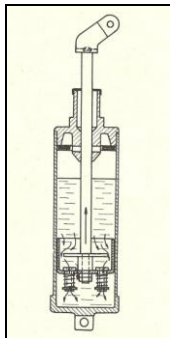
Beispiel: Rücklaufbremse der Astra-Werke AG, Chemnitz
