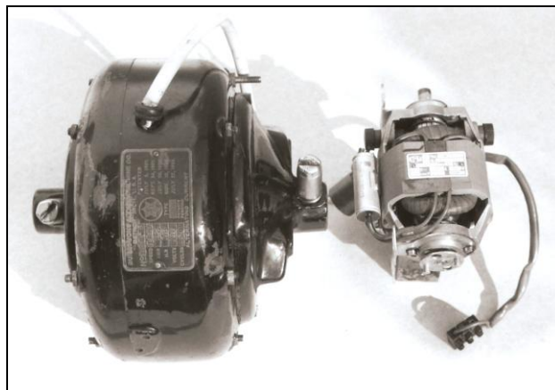
Abb. 8: Größenvergleich Antriebsmotoren
