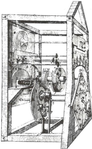
Abbildung von 1709 der Poleni-Rechenmaschine mit Gewichtsantrieb 22
