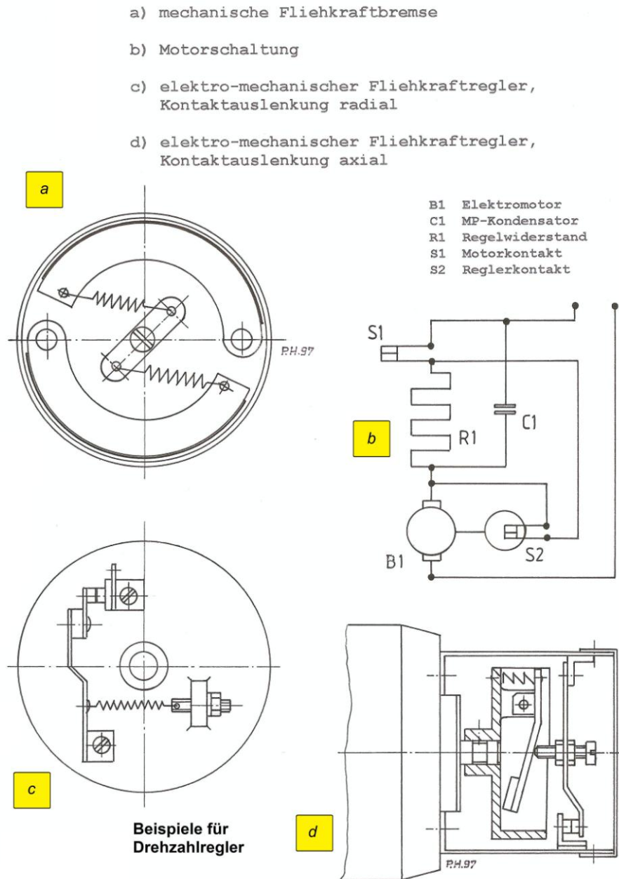
Abb. 9: Drehzahlregler
