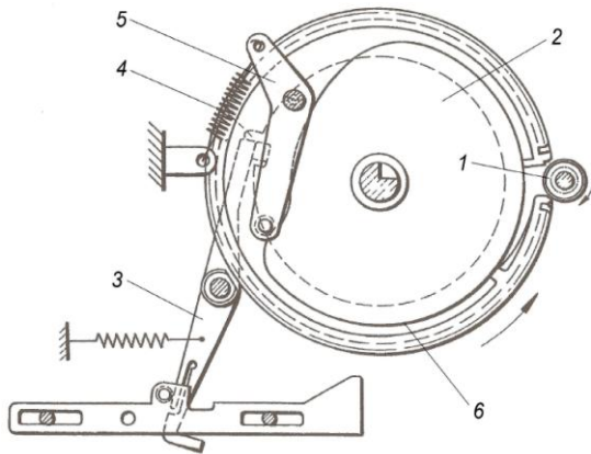
Beispiel einer temporären formschlüssigen Kupplungsverbindung: Olympia Modell AM
